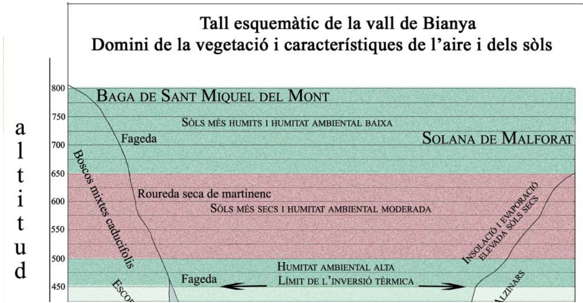
Figura 2: Tall esquemàtic de la Vall de Bianya: dominis de vegetació i característiques del sòl i de l'aire.
