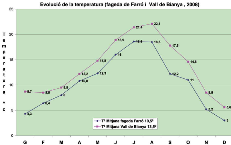
Figura 1: Comparativa de la temperatura (2008) entre la fageda de Farró (420) i la Vall de Bianya (440 m).
